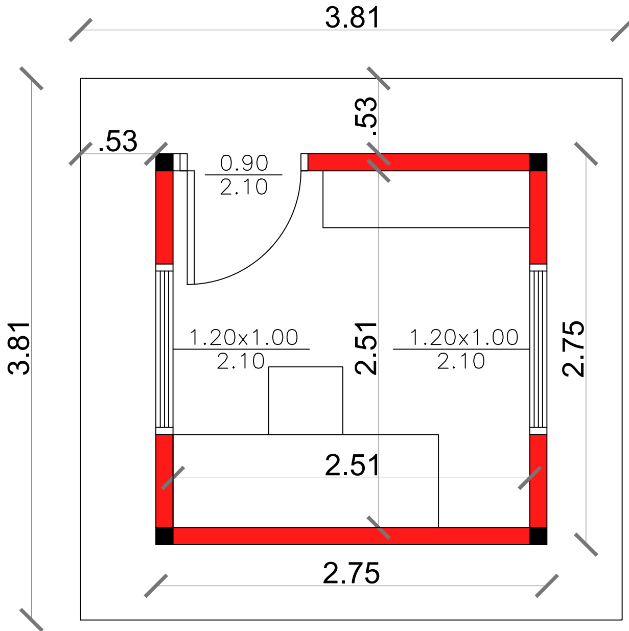
PLANTA GARITA ANEXO 5 ESC_1/50
